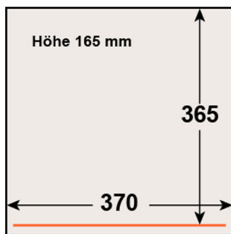
Schweissbalken 350 mm
