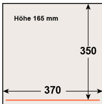
Schweissbalken 360 mm
